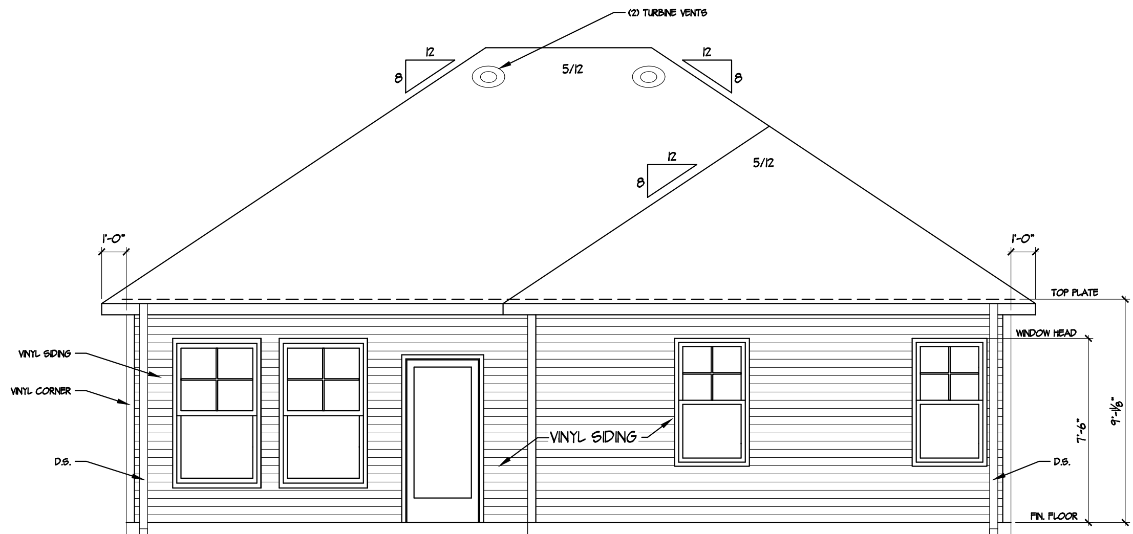
REAR ELEVATION SCALE: 1/8" = 1'-0"
